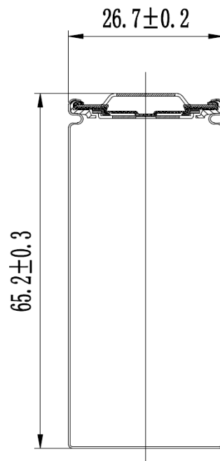
Figure 1 / 图 1 电芯外观尺寸
